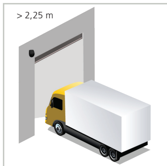
> 2,25 m La porte s'ouvre entièrement (détection de la hauteur - relais)
