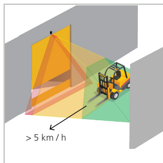
> 5 km / h La porte reste fermée.
